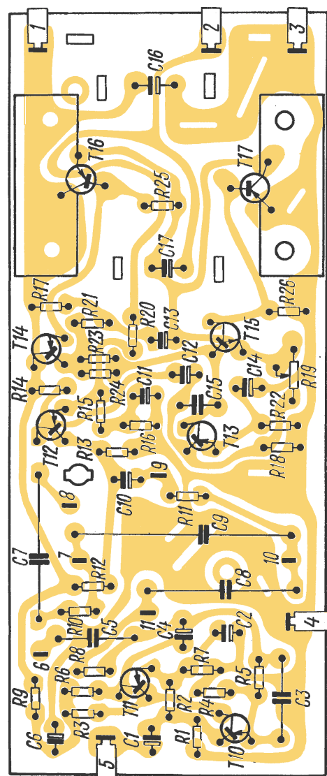
Рис. 12. Электромонтажная схема платы В4-П4 радиоприемника «Океан» На схеме не показаны экраны транзисторов Т3, Т4, Т5, Т8 и Т9 и положение подвижных ножей переключателя В1. Точки 20 и 21 платы соединены перемычкой
