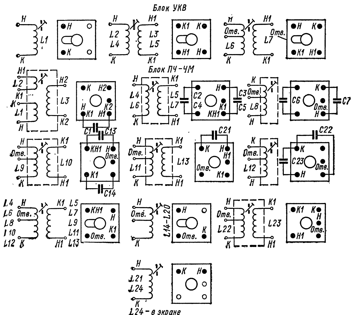
Рис. П-13. Распайка выводов катушек радиоприемника «Меридиан-202»
