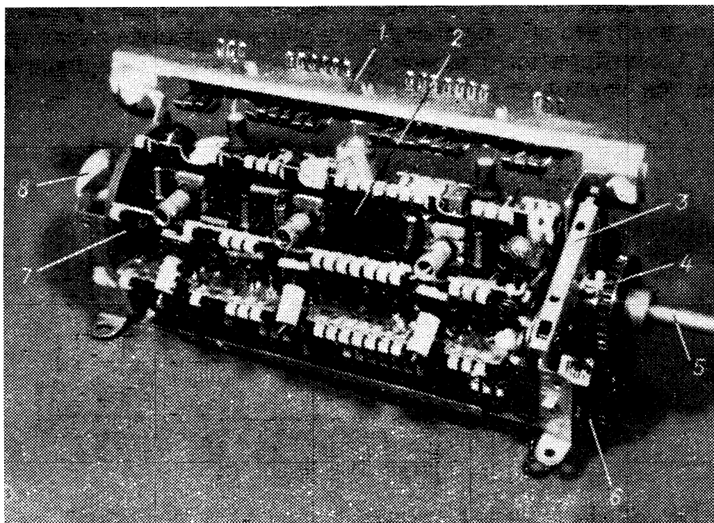
Рис. 48. Барабанный переключатель диапазонов радиоприемников «Океан» и «Океан-203»
