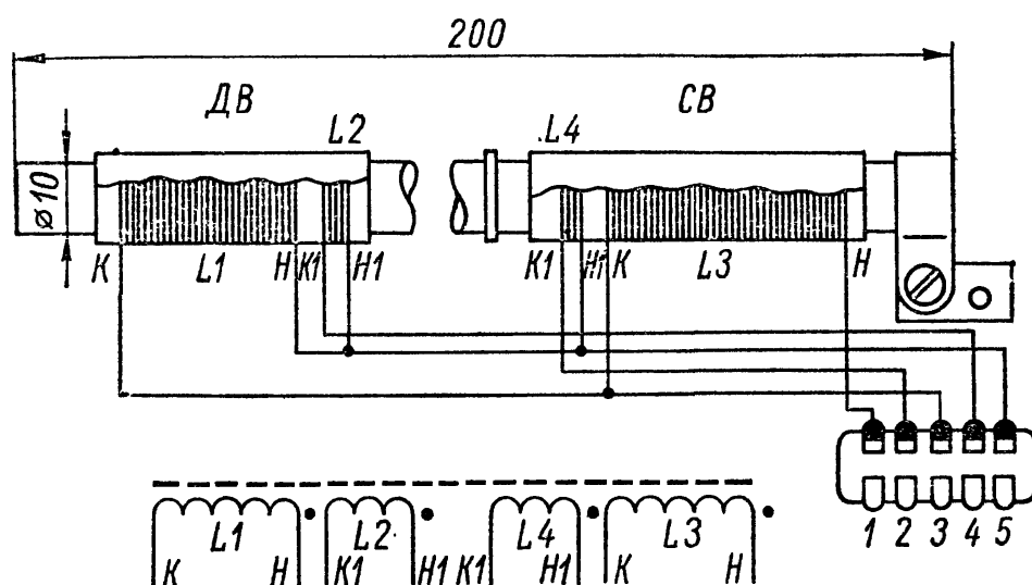
Рис. 49. Конструкция магнитной антенны радиоприемников «Океан» и «Океан-203»
