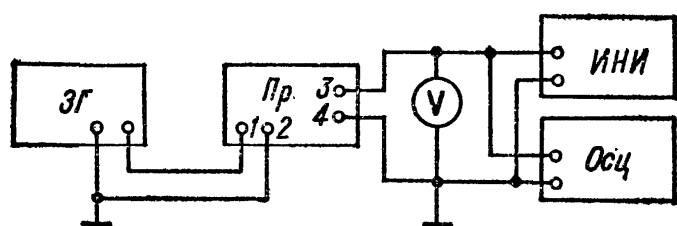
Рис. 69. Структурная схема настройки и проверки УНЧ приемников
