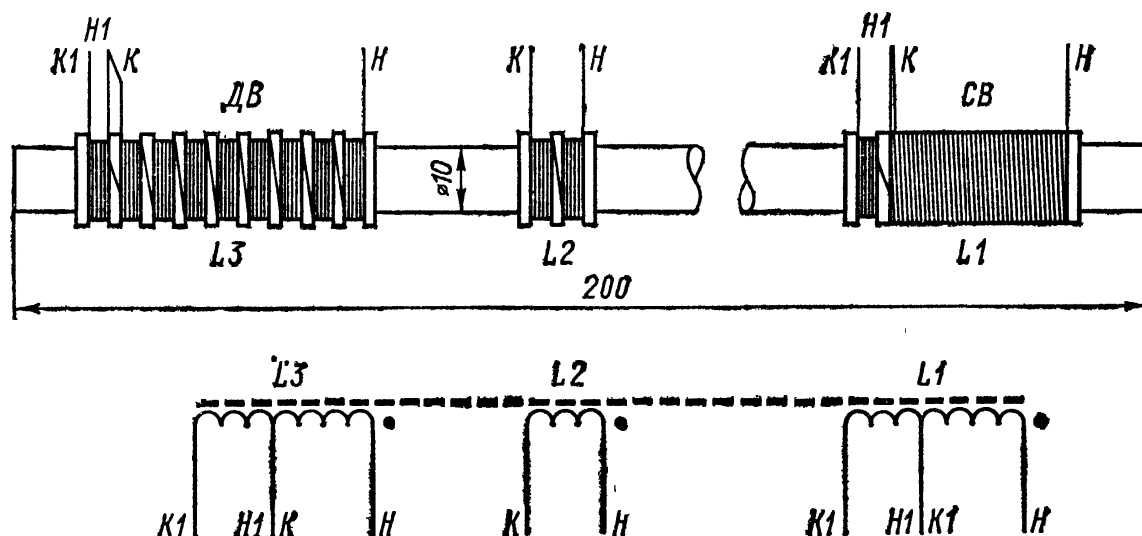
Рис. 60. Конструкция магнитной антенны радиоприемника «Украина-202»
