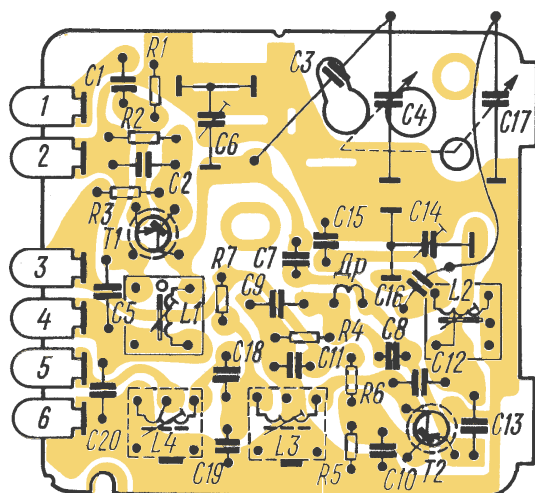
Рис. 11. Электромонтажная схема платы блока УКВ радиоприемника «Океан»
