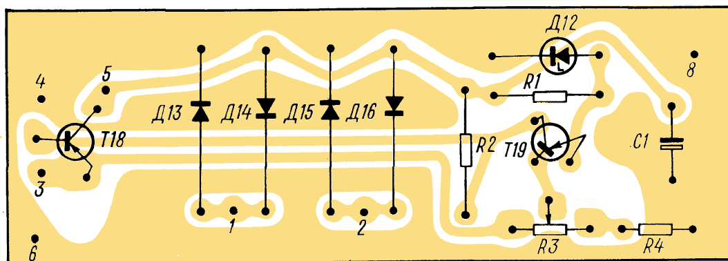
Рис. 22. Электромонтажная схема платы выпрямителя радиоприемника «Океан-205»
