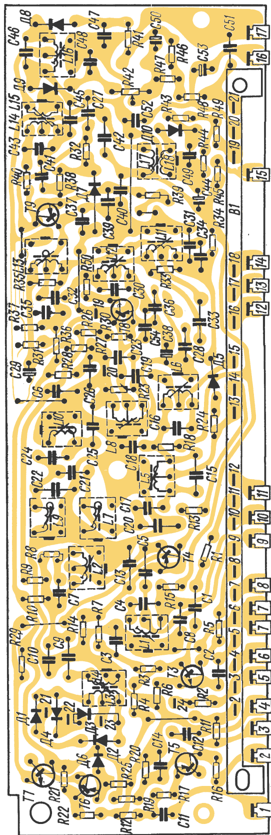
Рис. 12. Электромонтажная схема платы В4-П4 радиоприемника «Океан» На схеме не показаны экраны транзисторов Т3, Т4, Т5, Т8 и Т9 и положение подвижных ножей переключателя В1. Точки 20 и 21 платы соединены перемычкой
