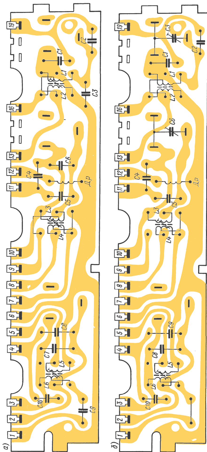
Рис. 15. Электромонтажные схемы планок диапазонов 25 м — П1, 31 м — П2, 41 м — П3, 49 м — П4(а); 50—75 м — П5(б) радиоприемника «Океан-203»
