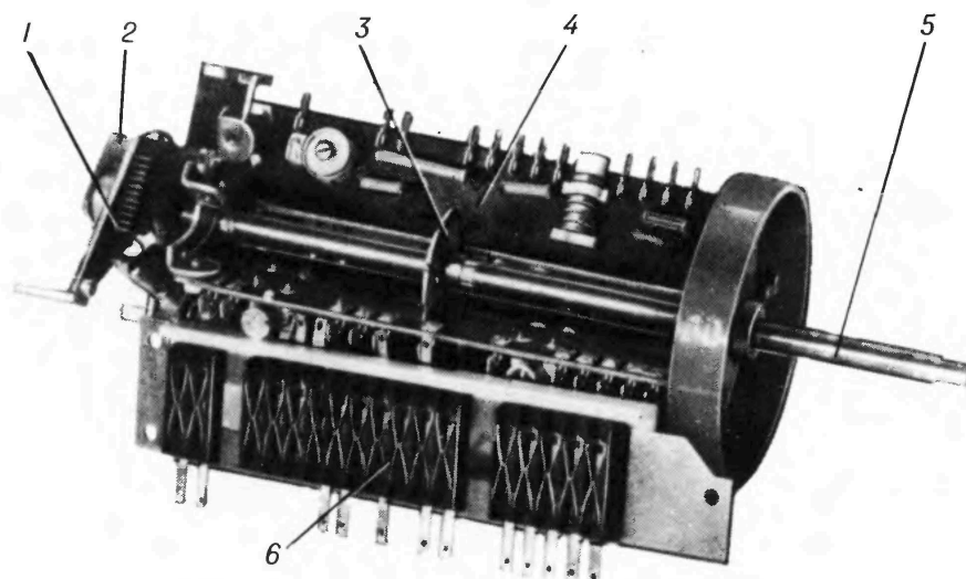
Рис. 56. Барабанный переключатель диапазонов радиоприемников «Спидола-207» и «Спидола-230»
