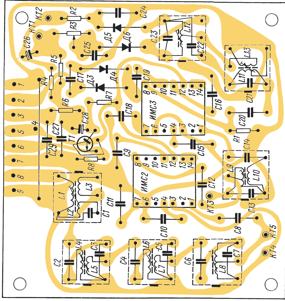
Рис. 33. Электромонтажная схема платы ПЧ-ЧМ радиоприемника «Меридиан-202»
