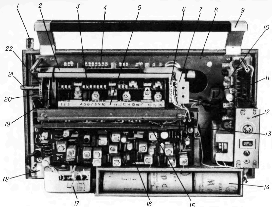
Рис. 53. Монтаж и размещение узлов радиоприемника «Океан-205»
