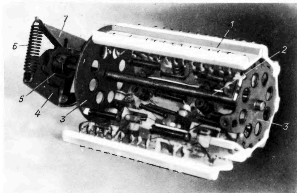
Рис. 39. Барабанный переключатель диапазонов радиоприемников «Спидола», «ВЭФ-Спидола» и «ВЭФ-Спидола-10»
