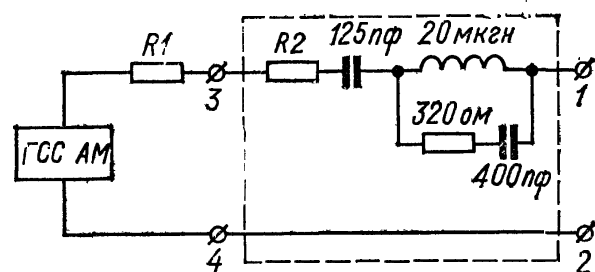
Рис. 75. Стандартный эквивалент антенны
