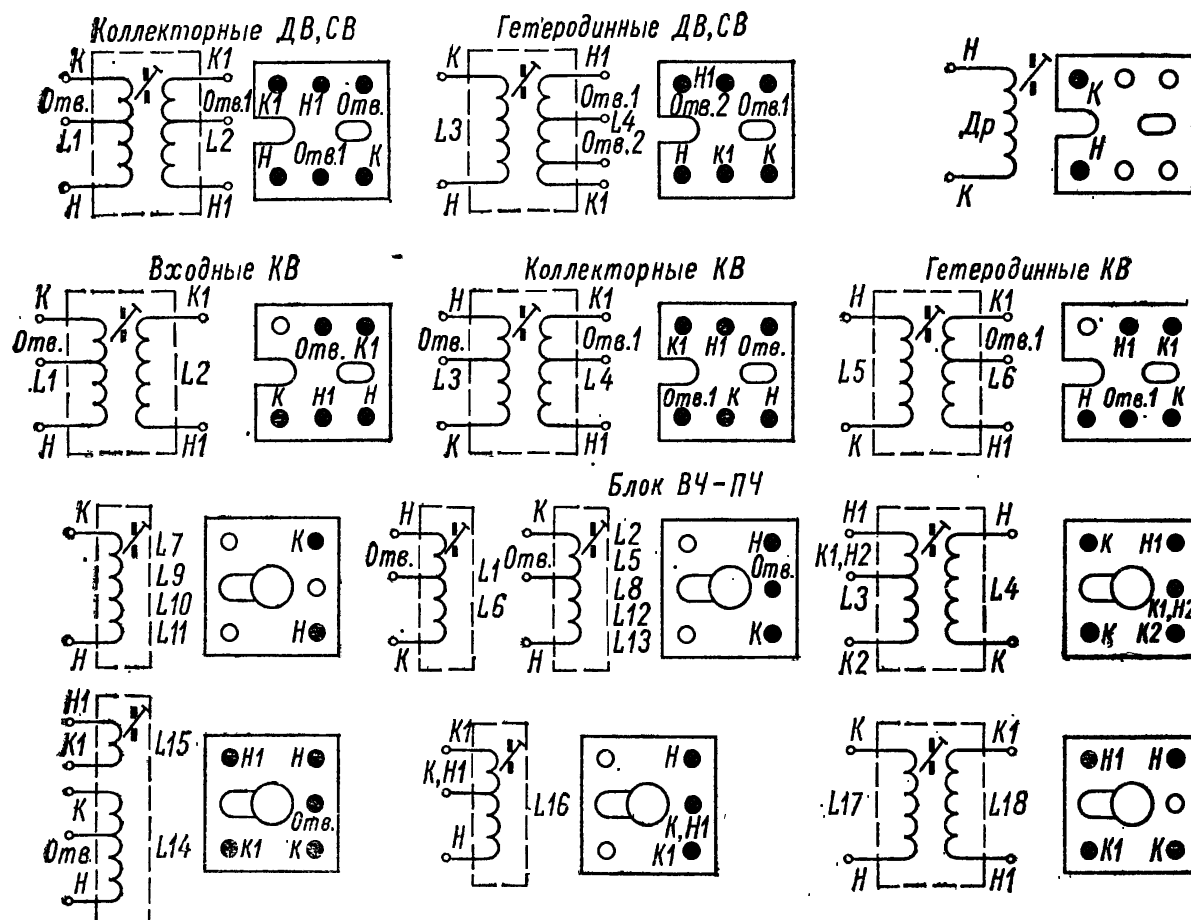
Рис. П-9. Распайка выводов катушек радиоприемников «Океан» и «Океан-203»
