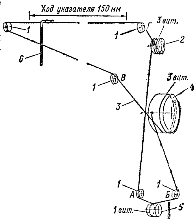
Рис. 57. Кинематическая схема верньерного устройства радиоприемника «Спидола-207»
