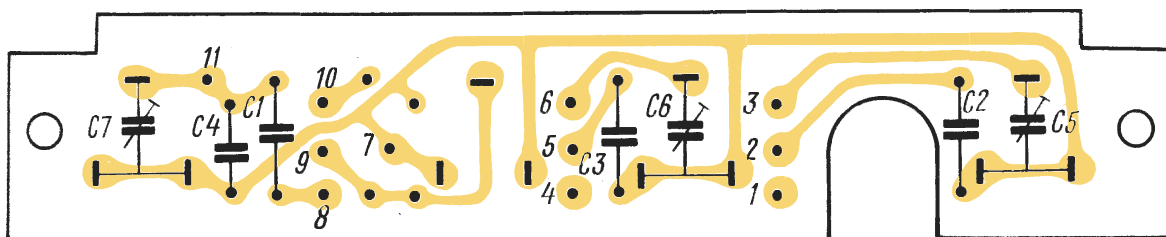
Рис. 35. Электромонтажная схема платы конденсаторов радиоприемника «Меридиан-202»
