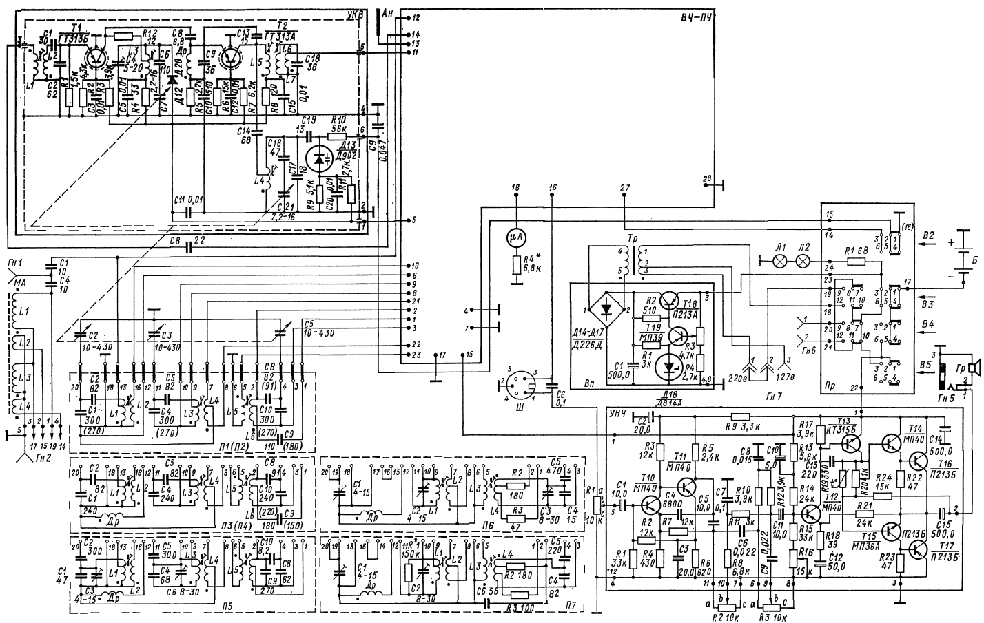
Рис. 19. Принципиальная схема радиоприемника «Океан-205»
