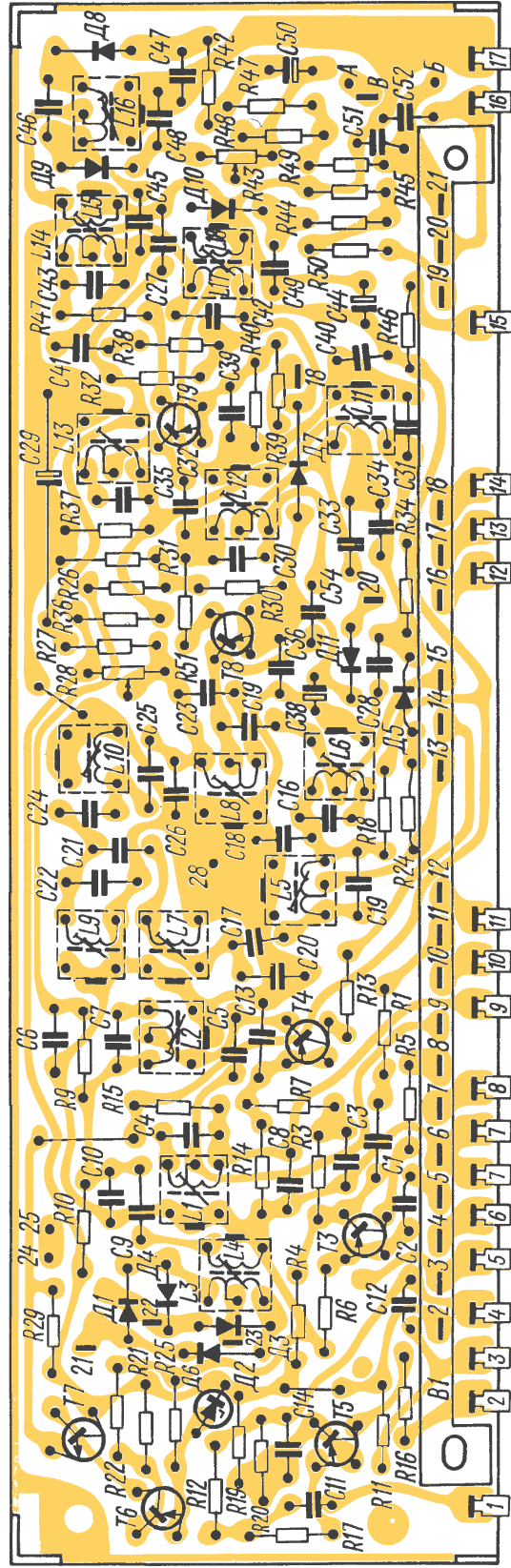
Рис. 17. Электромонтажная схема платы ВЧ-ПЧ радиоприемника «Океан-203» На схеме не показаны экраны транзисторов Т3, Т4, Т5, Т8 и Т9 и положение подвижных ножей переключателя В1
