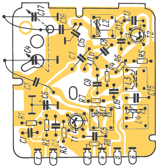
Рис. 16. Электромонтажная схема платы блока УКВ радиоприемника «Океан-203»
