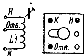
Рис. П-10. Распайка выводов катушки L1 блока УКВ радиоприемника «Океан-203»
