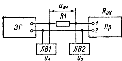
Рис. 70. Структурная схема измерения входного сопротивления УНЧ приемников
