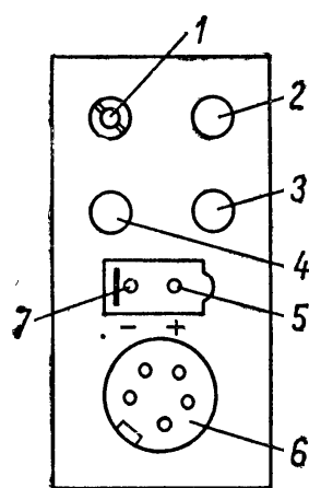
Рис. 47. Колодка внешних соединений радиоприемников «Океан» и «Океан-203»
