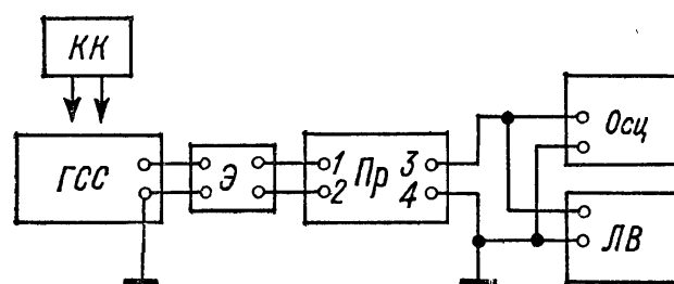
Рис. 76. Структурная схема проверки основных параметров приемников
