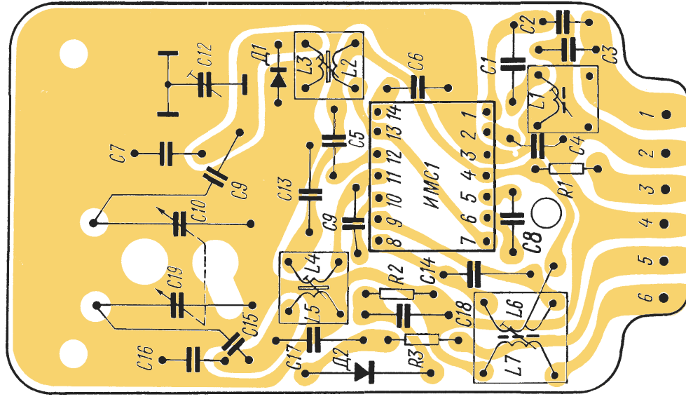
Рис. 32. Электромонтажная схема платы блока УКВ радиоприемника «Меридиан-202»
