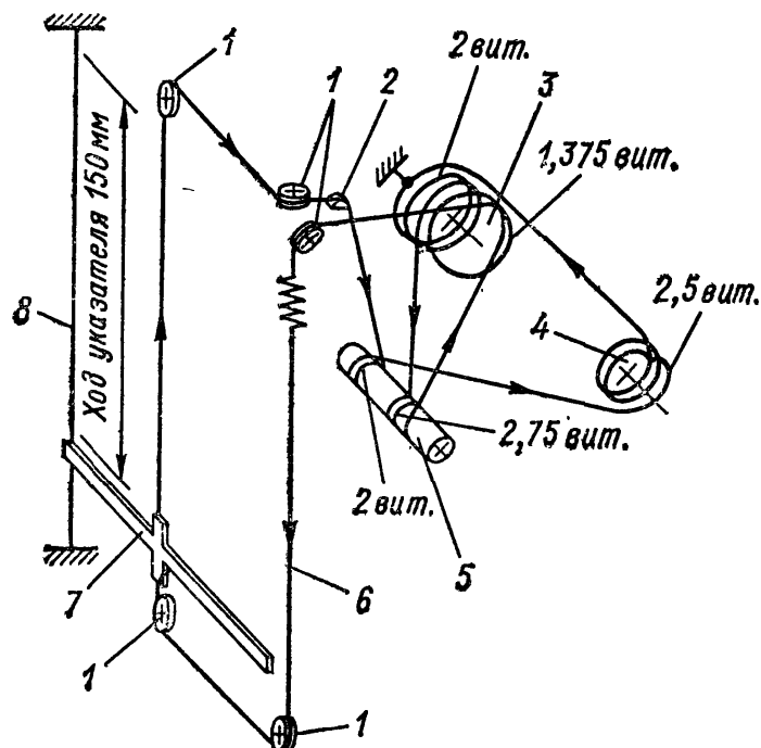
Рис. 61. Кинематическая схема верньерного устройства радиоприемника «Меридиан-202»
