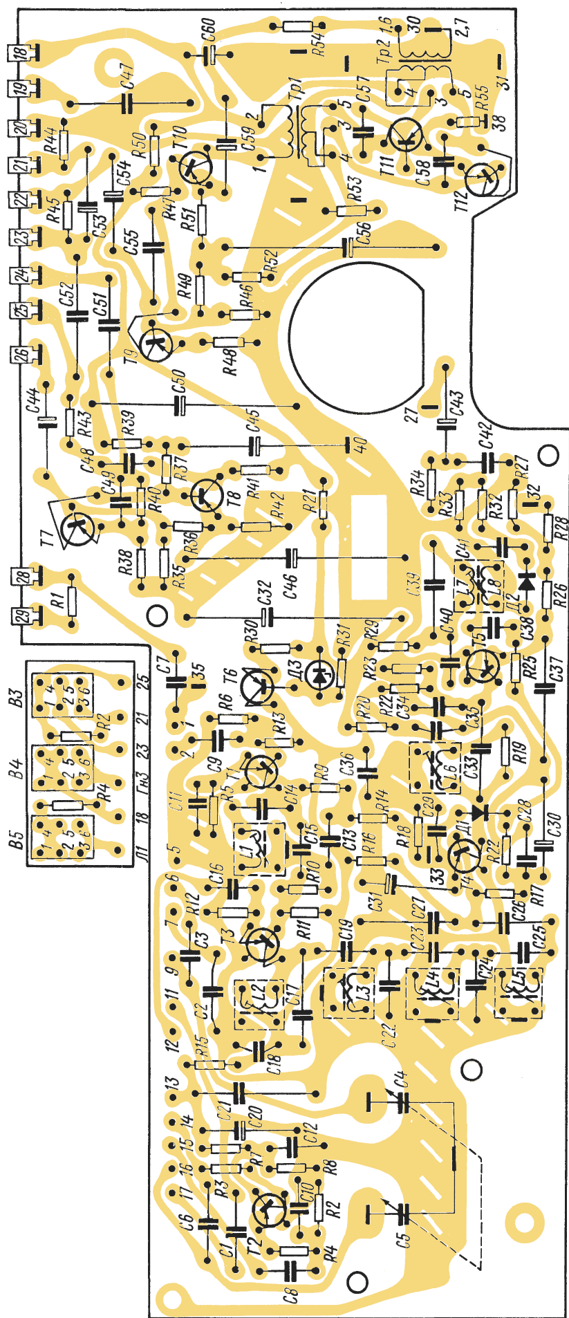
Рис. 30. Электромонтажная схема платы ПЧ-НЧ радиоприемника «Спидола-230»
