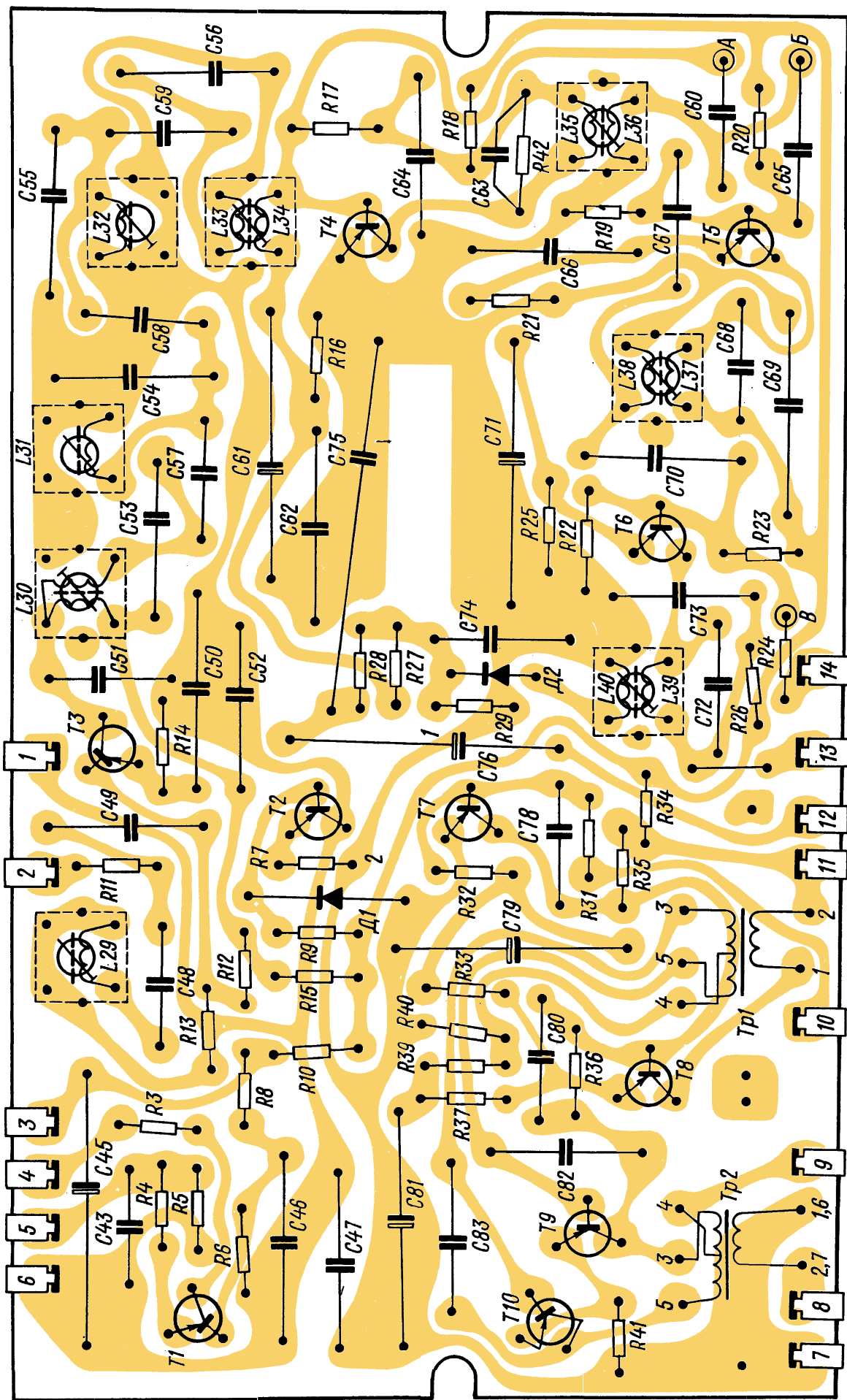
Рис. 2. Электромонтажная схема платы ПЧ-НЧ радиоприемников «Спидола», «ВЭФ-Спидола» и «ВЭФ-Спидола-10» Резистор R42 установлен со стороны фольги
