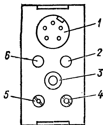
Рис. 59. Колодка внешних соединений радиоприемника «Меридиан-202»
