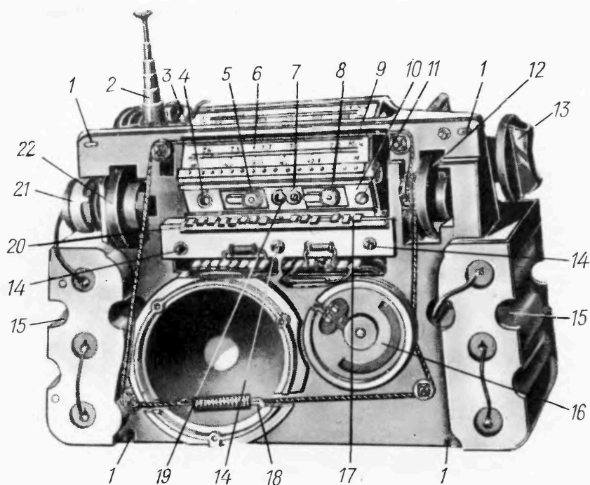
Рис. 38. Шасси радиоприемника «Спидола» в сборе (вид спереди)
