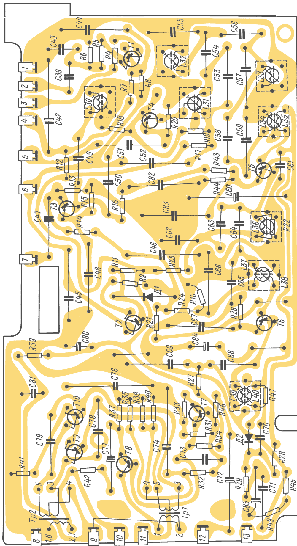
Рис. 6. Электромонтажная схема платы ПЧ-НЧ радиоприемников «ВЭФ-12», «ВЭФ-201» и «ВЭФ-202» Резисторы R10, R22 и R47 установлены со стороны фольги
