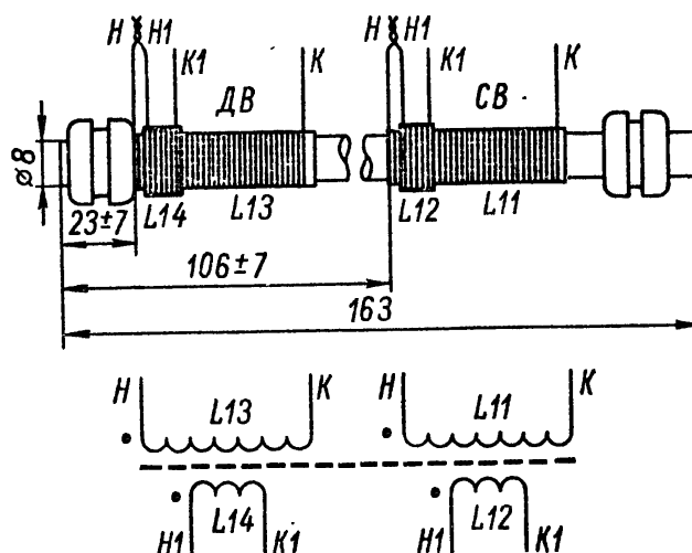
Рис. 40. Конструкция магнитной антенны радиоприемников «Спидола», «ВЭФ-Спидола» и «ВЭФ-Спидола-10»
