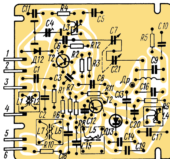
Рис. 20. Электромонтажная схема платы блока УКВ радиоприемника «Океан-205»
