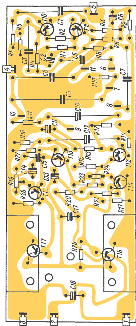
Рис. 18. Электромонтажная схема платы УНЧ радиоприемника «Океан-203»
