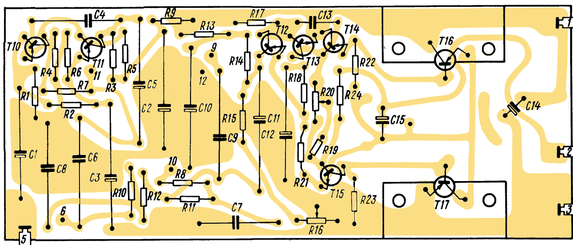
Рис. 21. Электромонтажная схема платы УНЧ радиоприемника «Океан-205»
