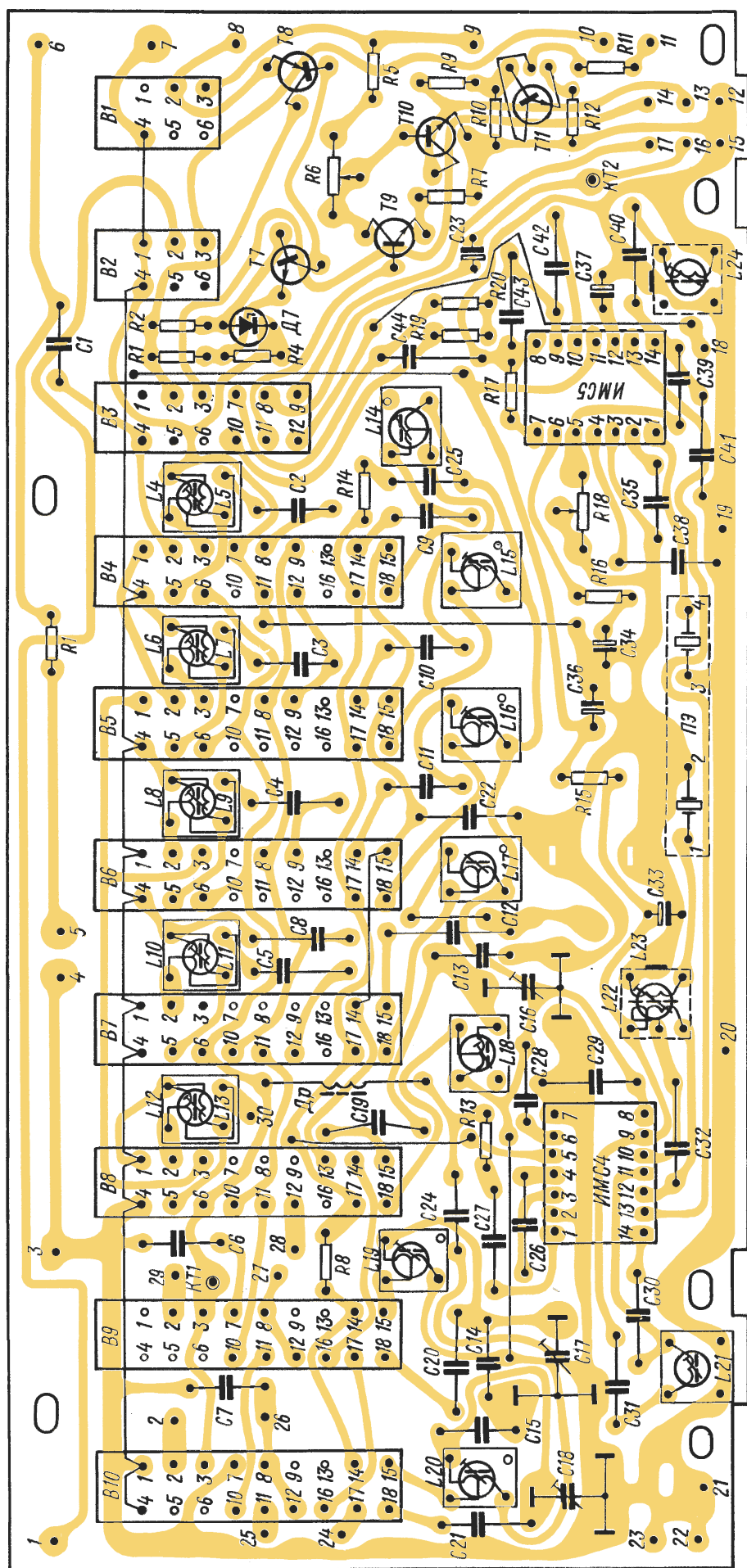
Рис. 34. Электромонтажная схема платы ВЧ-ПЧ АМ радиоприемника «Меридиан-202»
