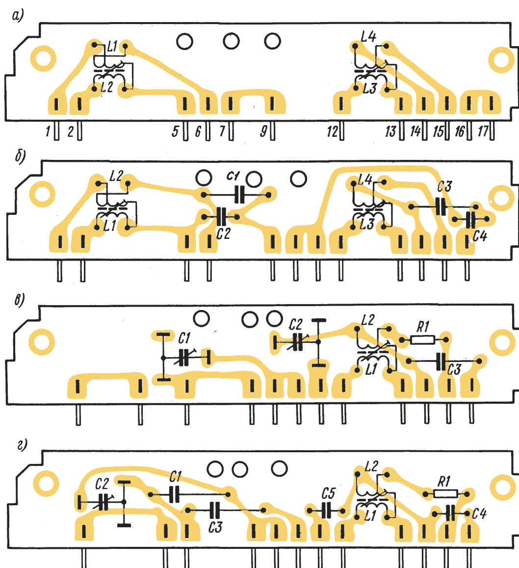
Рис. 27. Электроmontажные схемы планок диапазонов 25 м — П1, 31 м — П2, 41 м — П3, 49 м — П4(а); 52—75 м — П5(б); СВ — П6(в); ДВ — П7(г) радиоприемников «Спидола-207» и «Спидо- ла-230»
