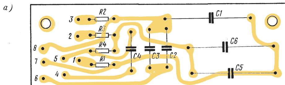
Рис. 35. Электромонтажная схема платы конденсаторов радиоприемника «Меридиан-202»
