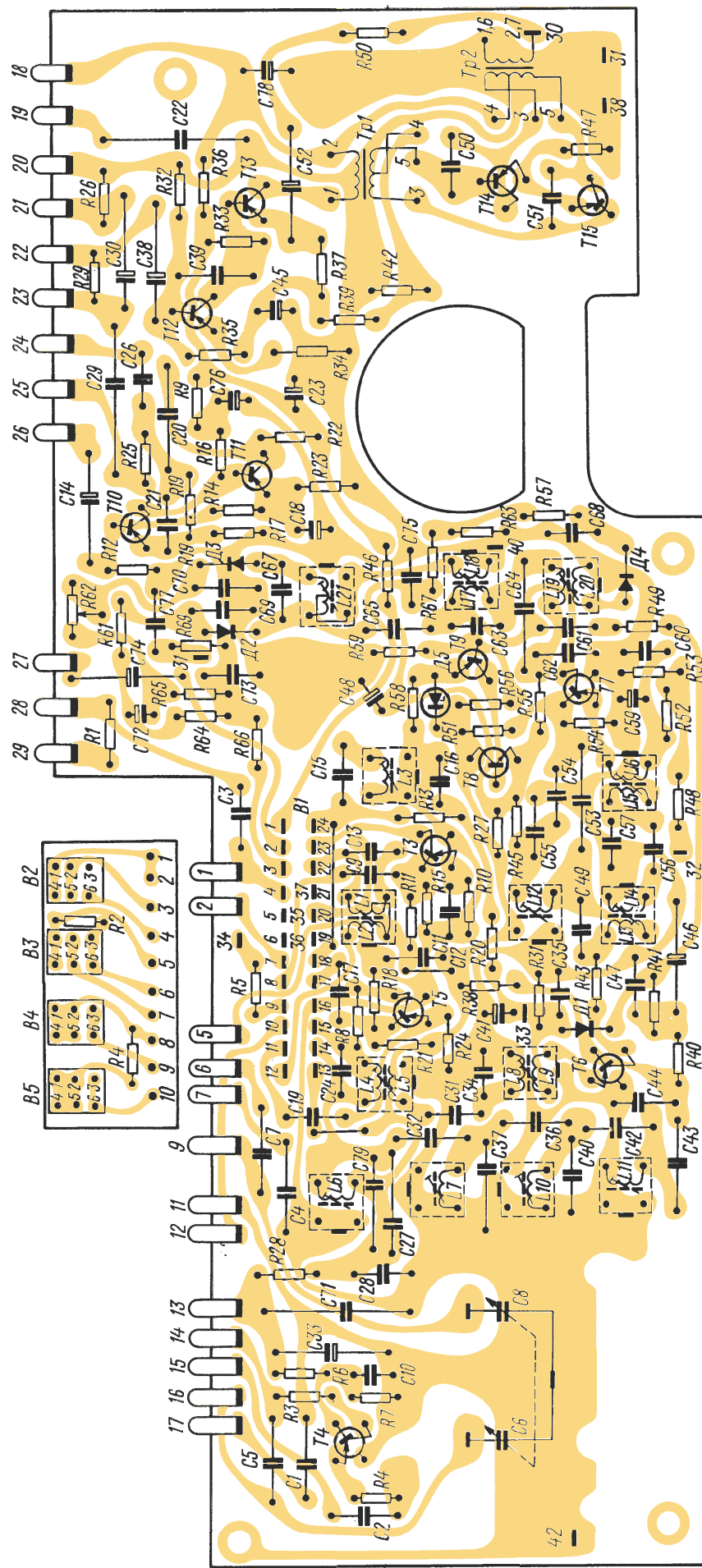
Рис. 28. Электромонтажная схема платы ПЧ-НЧ радиоприемника «Спидола-207» Экраны транзисторов Т3 — Т7 показаны условно. Положения подвижных ножек переключателей В1 — В5 не показаны
