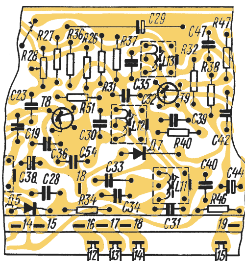
Рис. 25. Участок электроmontажной схемы платы ВЧ-ПЧ радиоприемника «Океан-205» с измененной печатью
