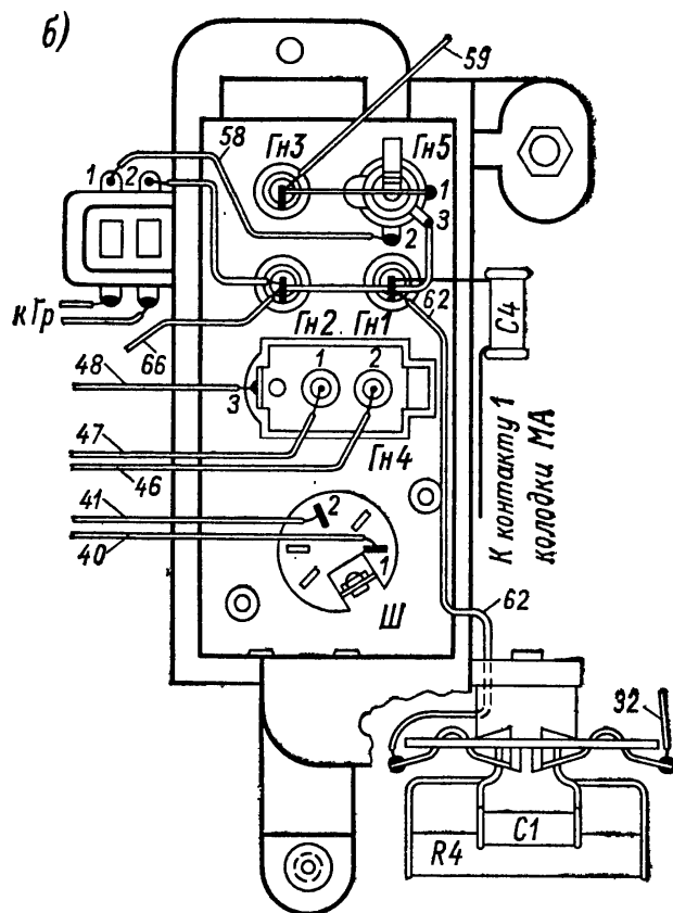
Рис. 51, б. Схема колодки внешних соединений радиоприемника «Океан»
