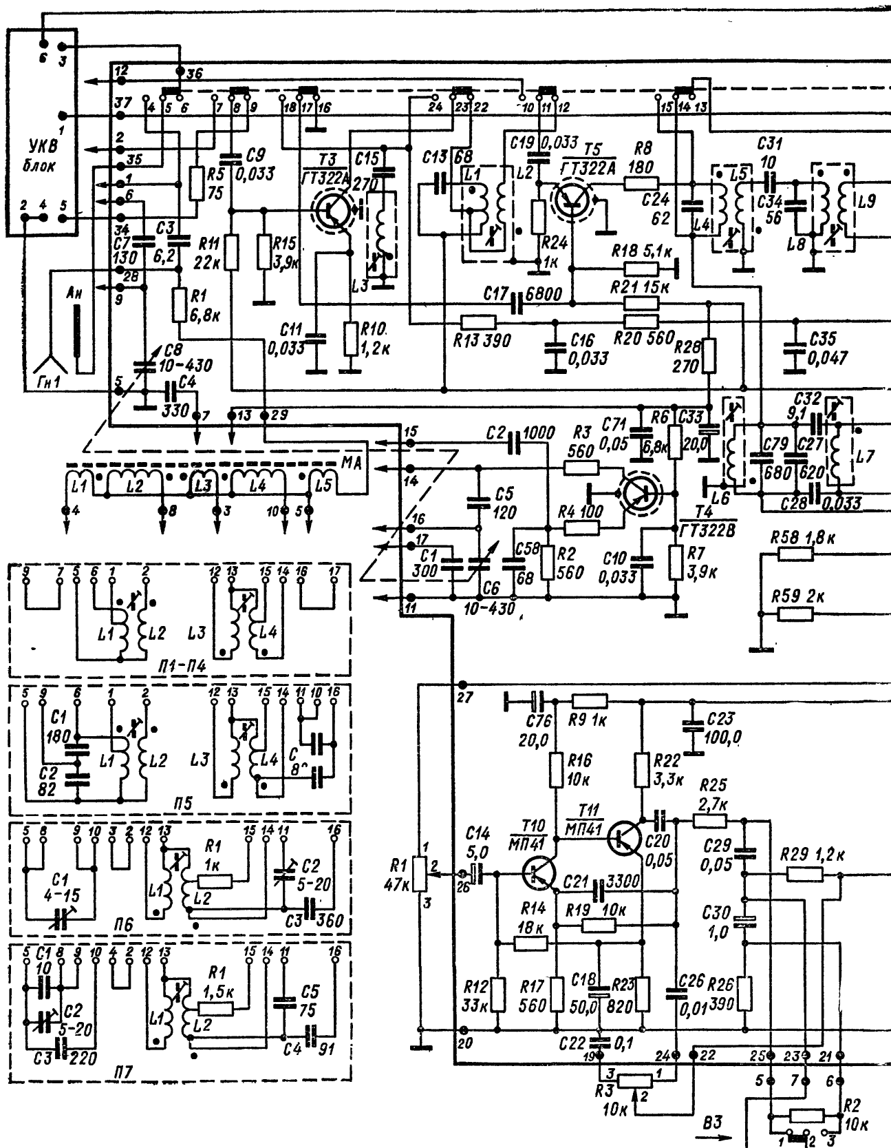
Рис. 26. Принципиальная схема
