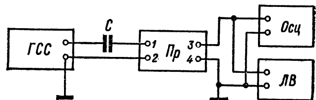
Рис. 71. Структурная схема настройки и проверки УПЧ приемников
